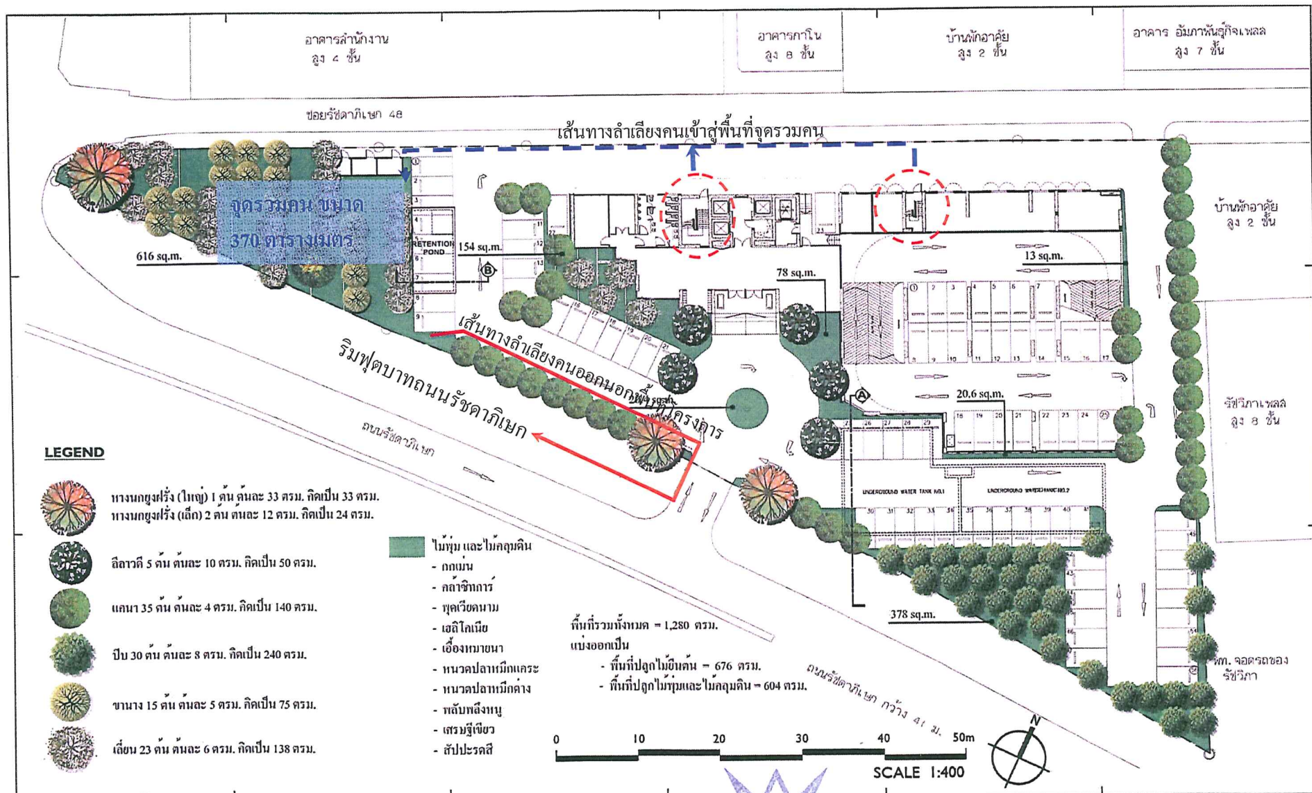
รูปที่ 7 ตำแหน่งจุดรวมคนและเส้นทางอพยพหนีไฟ
