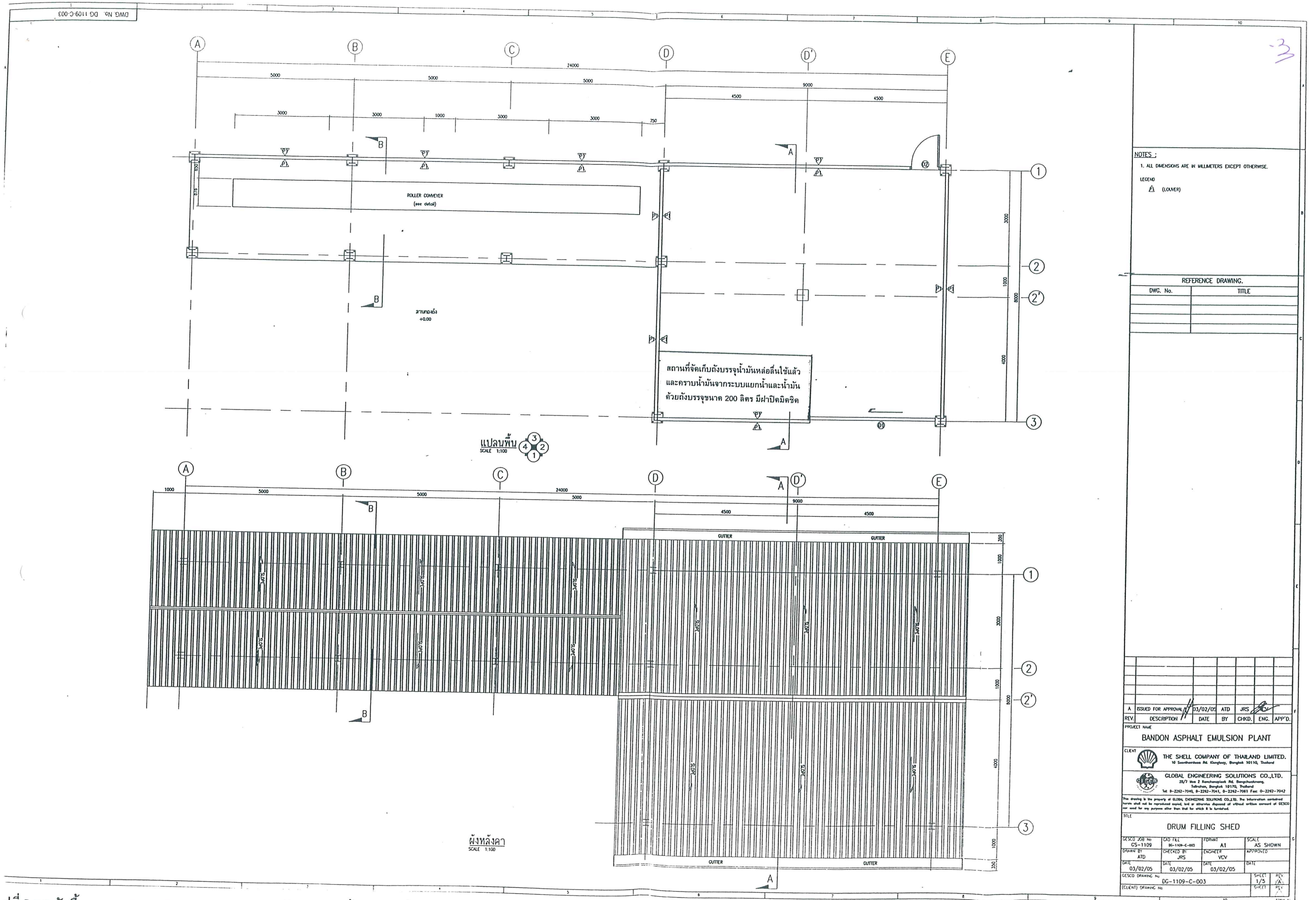
ปที่ 5.2-3 ผังพื้นอาคาร Drum Filling แสดงตำแหน่งเก็บถังบรรจุน้ำมันหล่อลื่นใช้แล้ว
