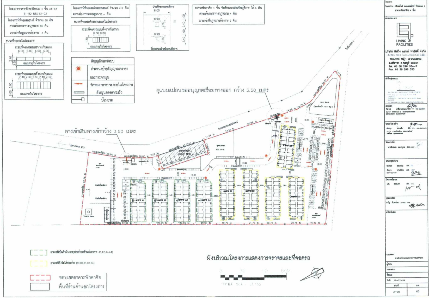
รูปที่ 9 ผังบริเวณโครงการแสดงการจราจรและที่จอดรถ
