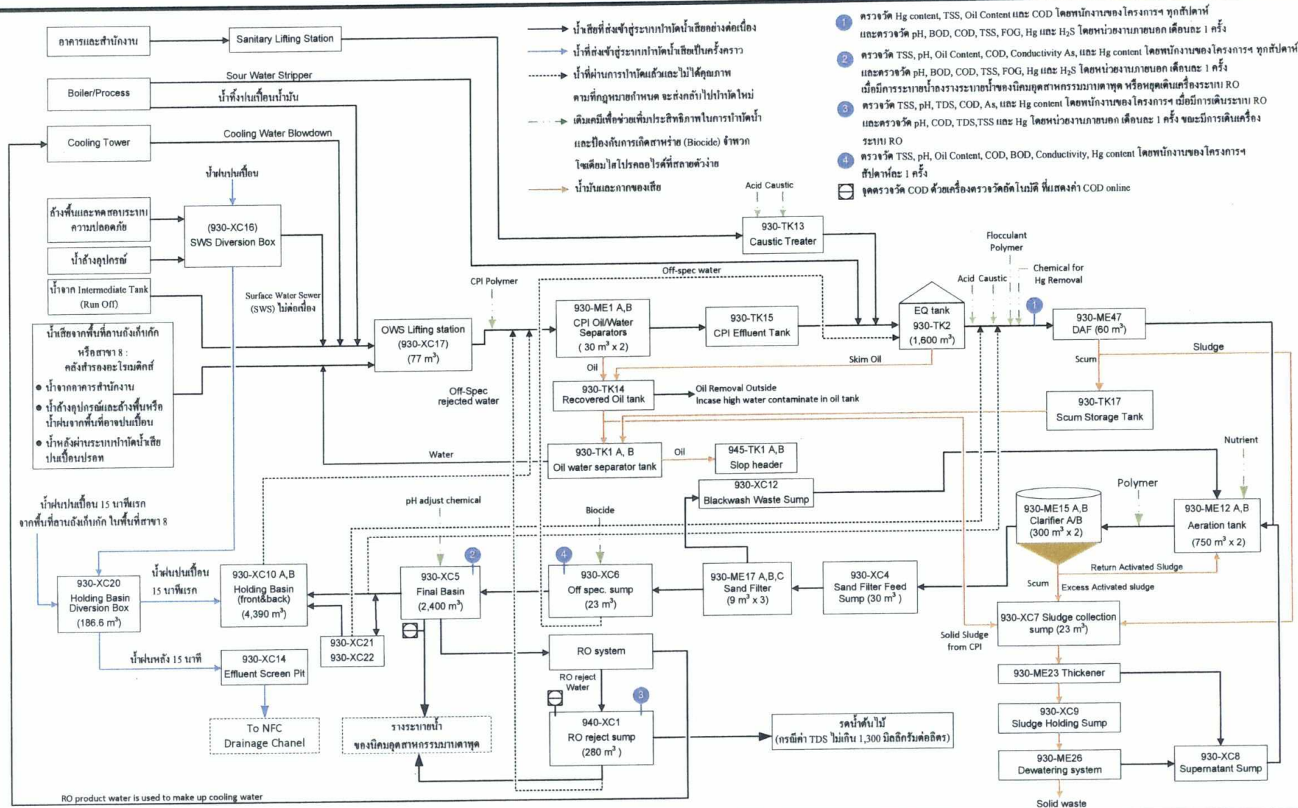
รูปที่ 2 แผนผังตอนการทำงานระบบบำบัดน้ำเสีย โครงการโรงผลิตสารอะโรเมติกส์ หน่วยที่ 1 (ส่วนขยาย ครั้งที่ 4) บริษัท พีทีที โกลบอล เคมิคอล จำกัด (มหาชน)
