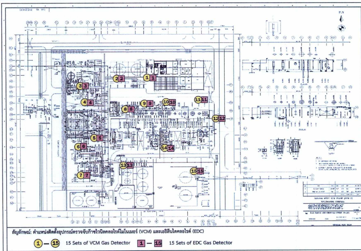
รูปที่ 27 ตำแหน่งติดตั้งอุปกรณ์ตรวจก๊าซไวโนลคลอไรด์โมโนเมอร์ (VCM) และเออีซีนไคคลอไรด์ (EDC) บริเวณโรงงาน VCM 2
