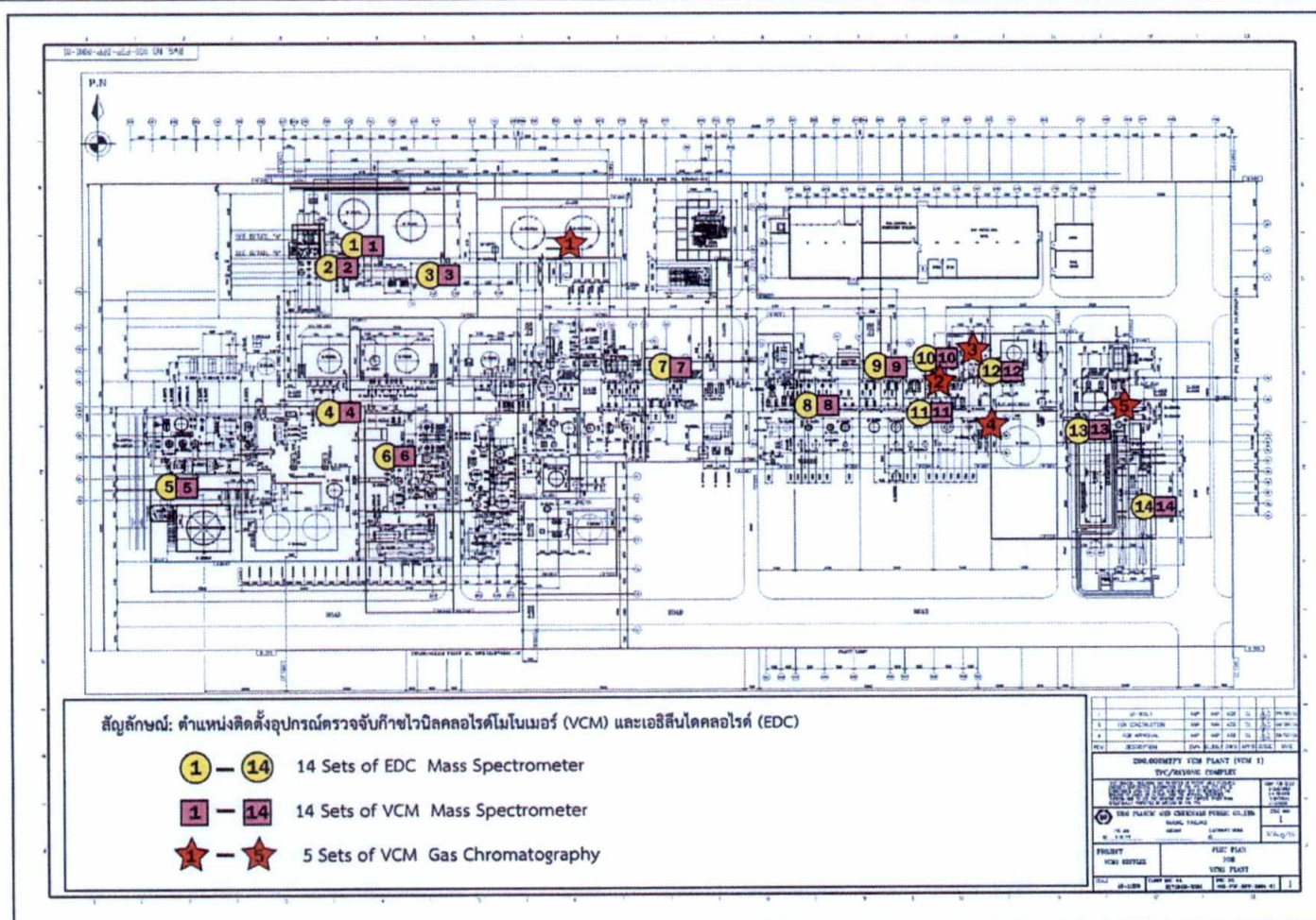
รูปที่ 26 ตำแหน่งติดตั้งอุปกรณ์ตรวจจับก๊าซไว้นิลคโครไรต์โมโนเมอร์ (VCM) และเอธิซีนไดคลอไรด์ (EDC) บริเวณโรงงาน VCM 1
