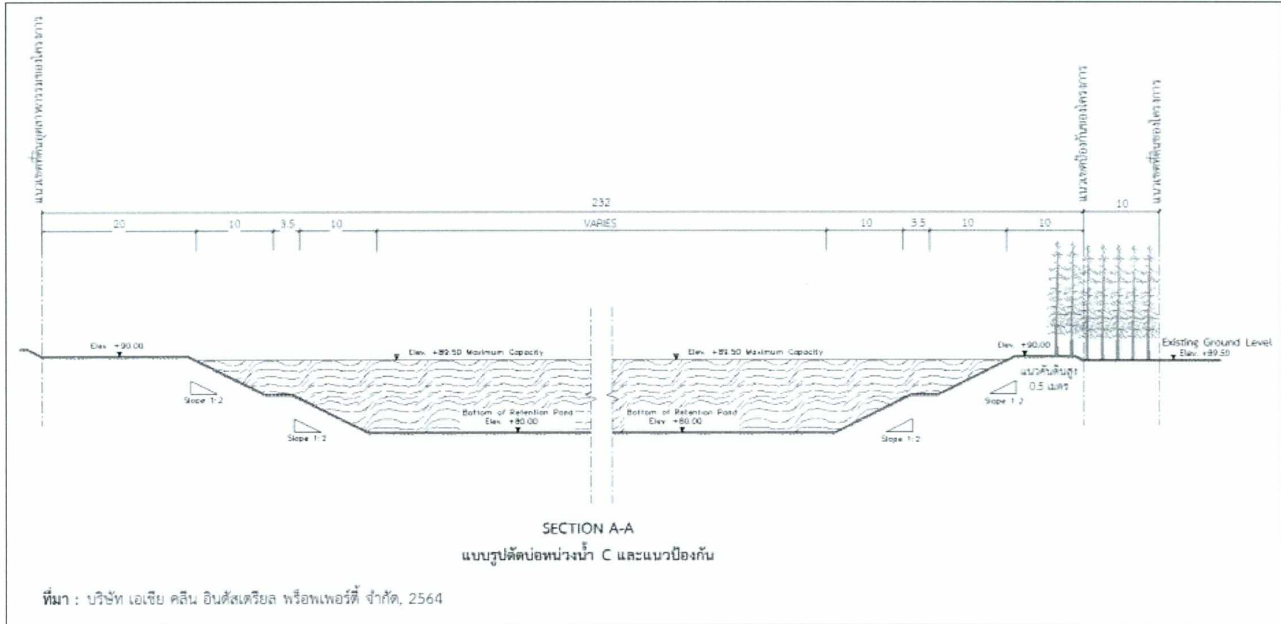
รูปที่ 4 รูปตัดขวาง (Cross Section) ของพื้นที่สีเขียวที่ใช้เป็นแนวป้องกันของโครงการ (ต่อ)
