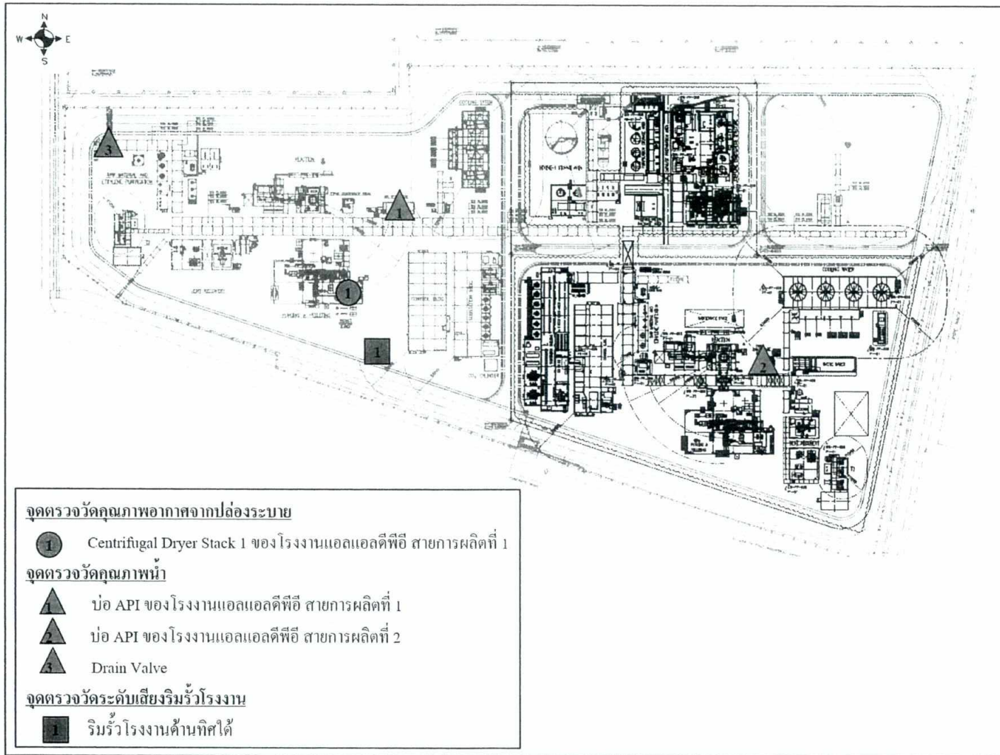
รูปที่ 6 จุดตรวจวัดคุณภาพอากาศจากปล่องระบาย คุณภาพน้ำ และระดับเสียงริมรั้วโรงงาน
