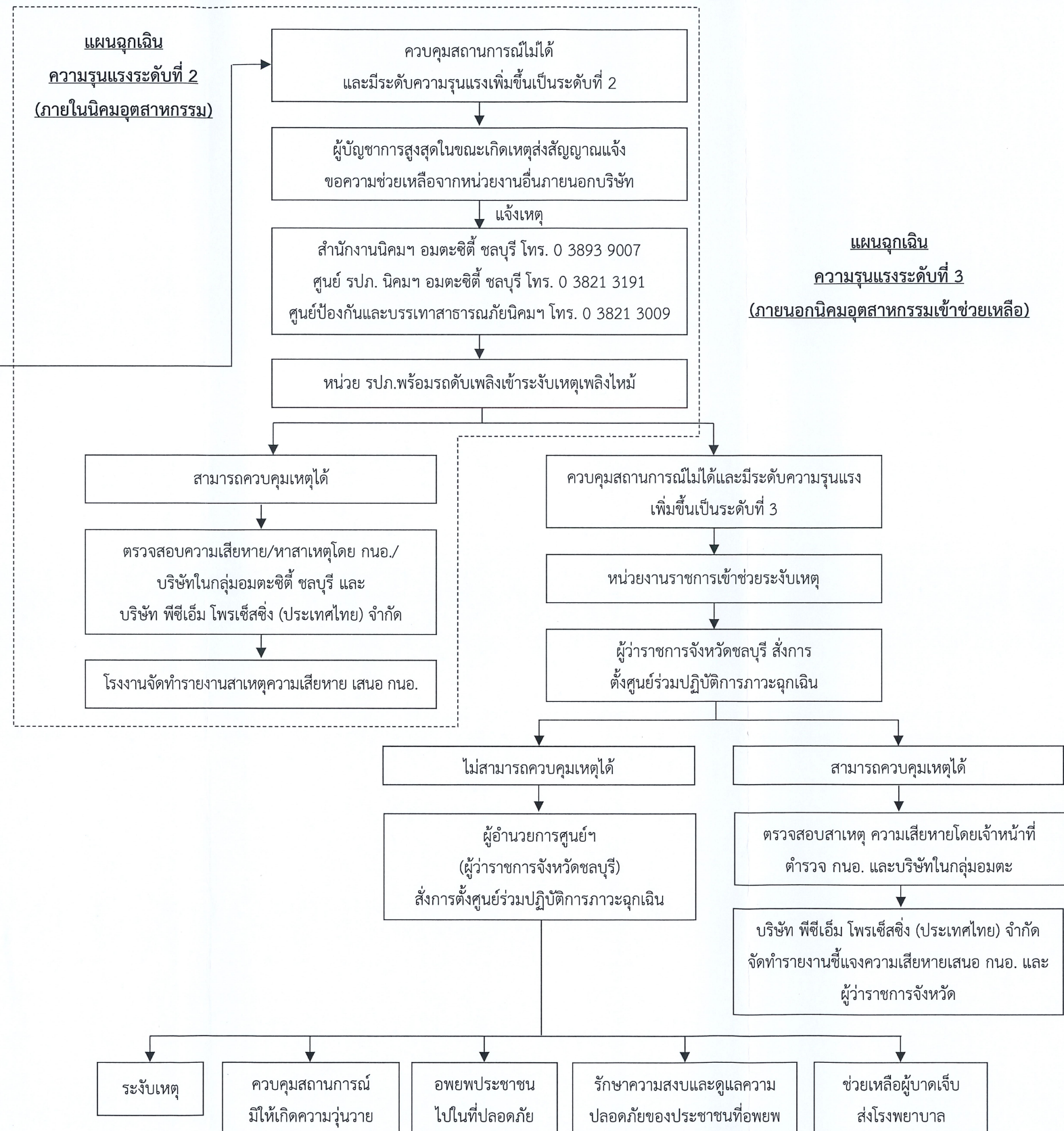
รูปที่ 4 ผังการสื่อสาร ประสานงาน และแผนฉุกเฉินของโครงการที่เชื่อมโยงกับนิคมอุตสาหกรรมอมตะซิตี้ ชลบุรี
