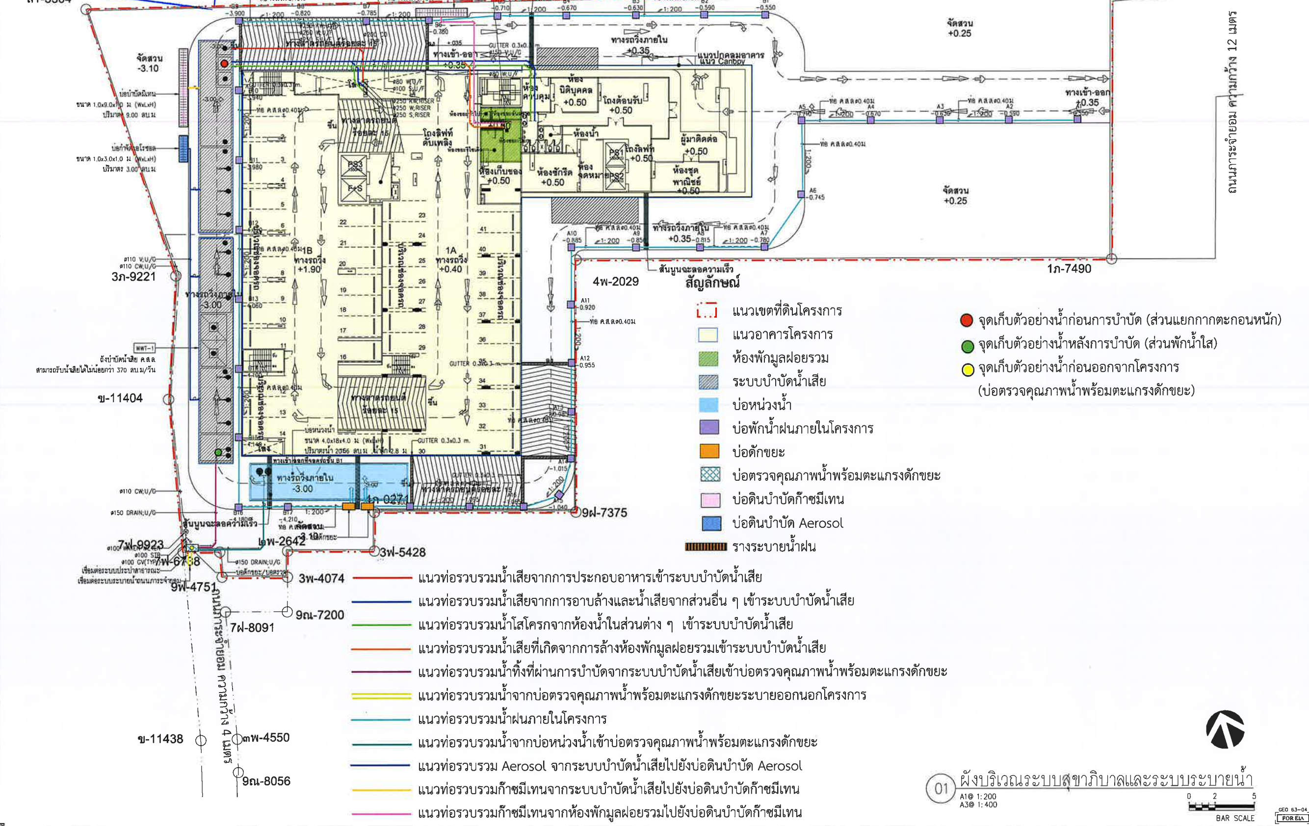
รูปที่ 6 ผังระบบระบายน้ำของโครงการ
