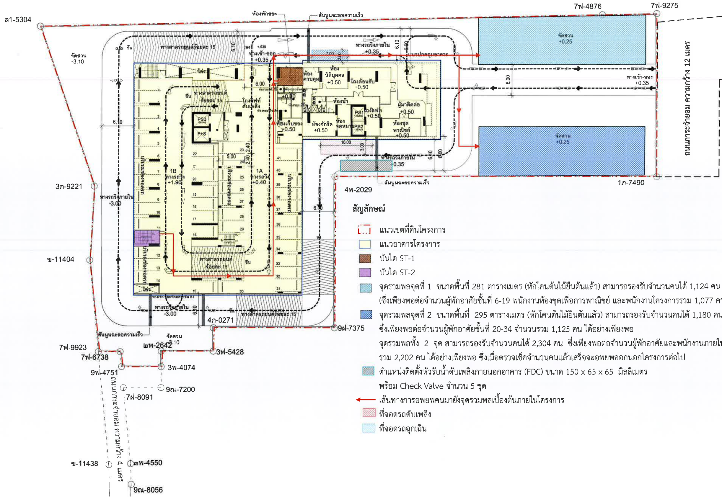
รูปที่ 7 ตำแหน่งบันไดที่ใช้หนีไฟ และเส้นทางอพยพคนมายังจุดรวมพลภายในโครงการ
