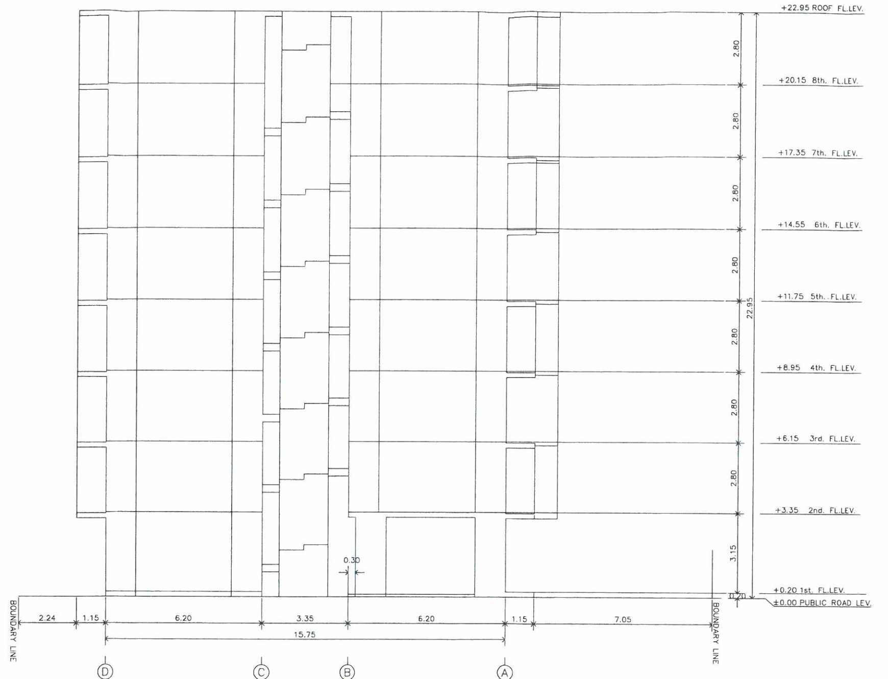
ELEVATION 2
