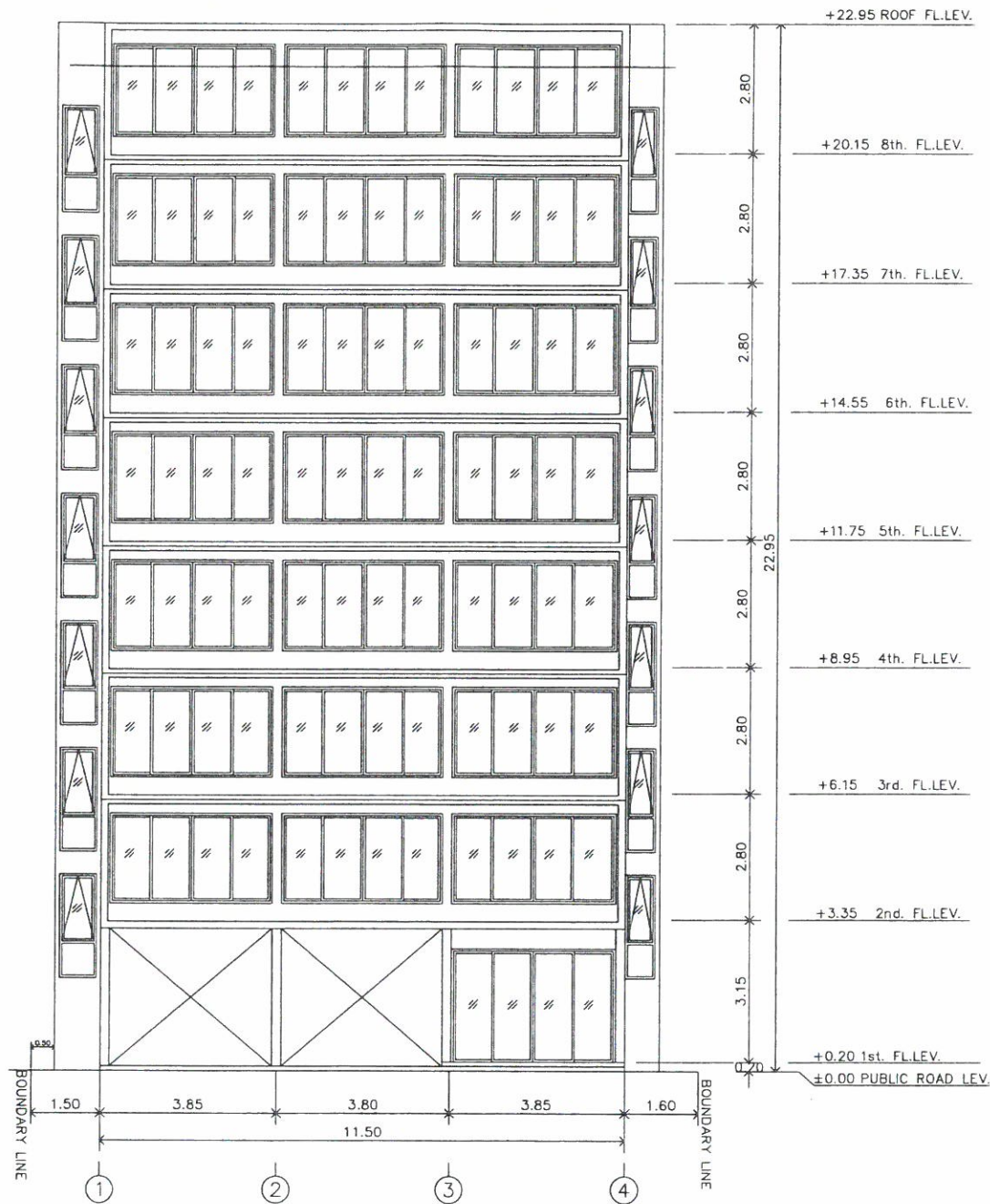
ELEVATION 1
