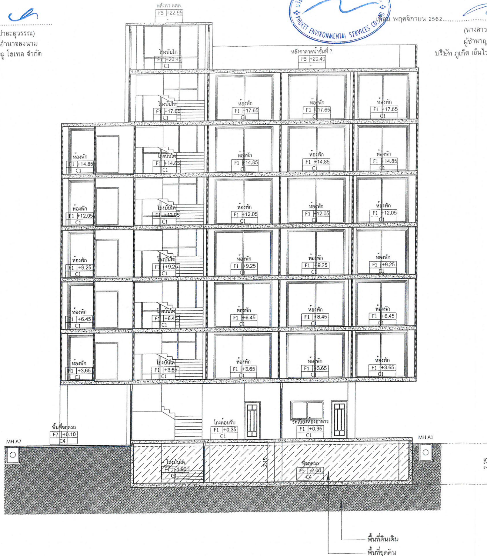
รูปตัดแสดงความลึกพื้นที่ขุดดิน SCALE A3-1:125
