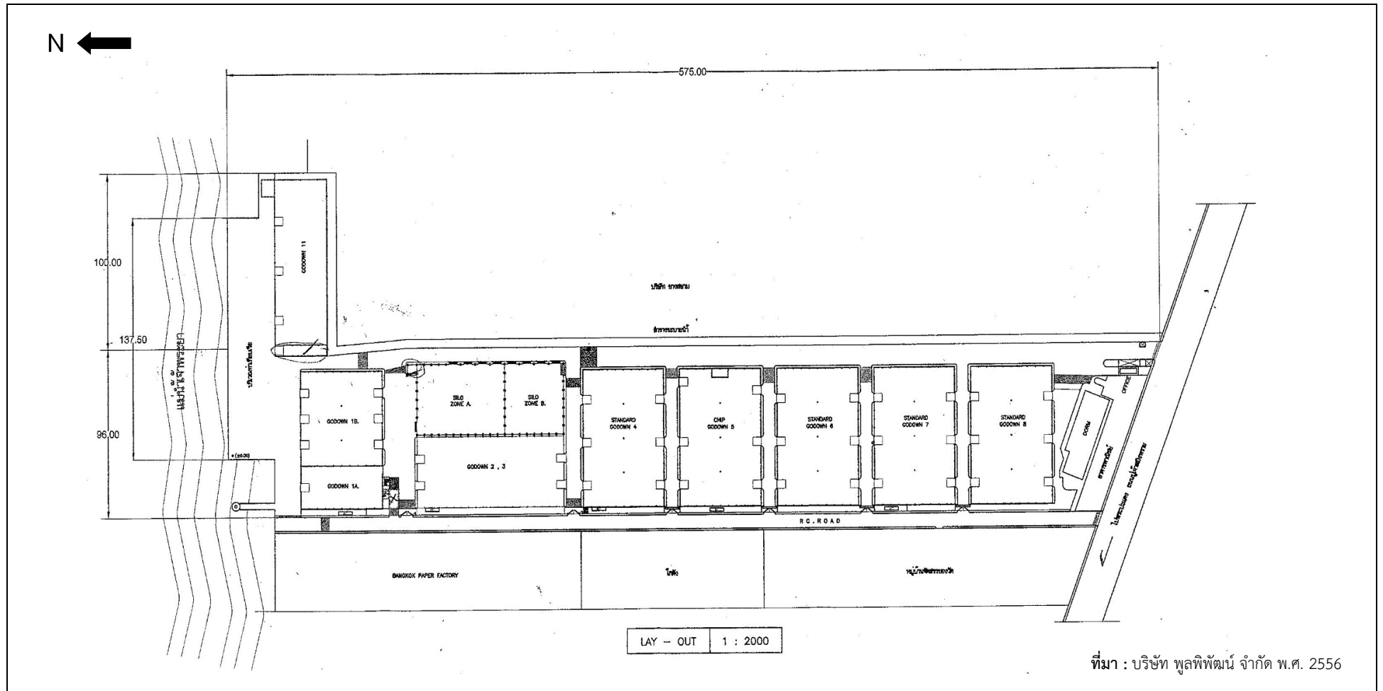
รูปที่ 1-2 แผนผังแสดงการใช้ประโยชน์ที่ดินของโครงการท่าเทียบเรือ บริษัท พูลพิพัฒน์ จำกัด
