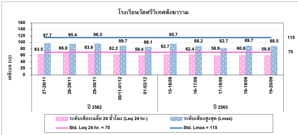
รูปที่ 4.2-1 กราฟเปรียบเทียบผลการตรวจวัดระดับเสียงโดยทั่วไป ระหว่างปี 2562-2563
