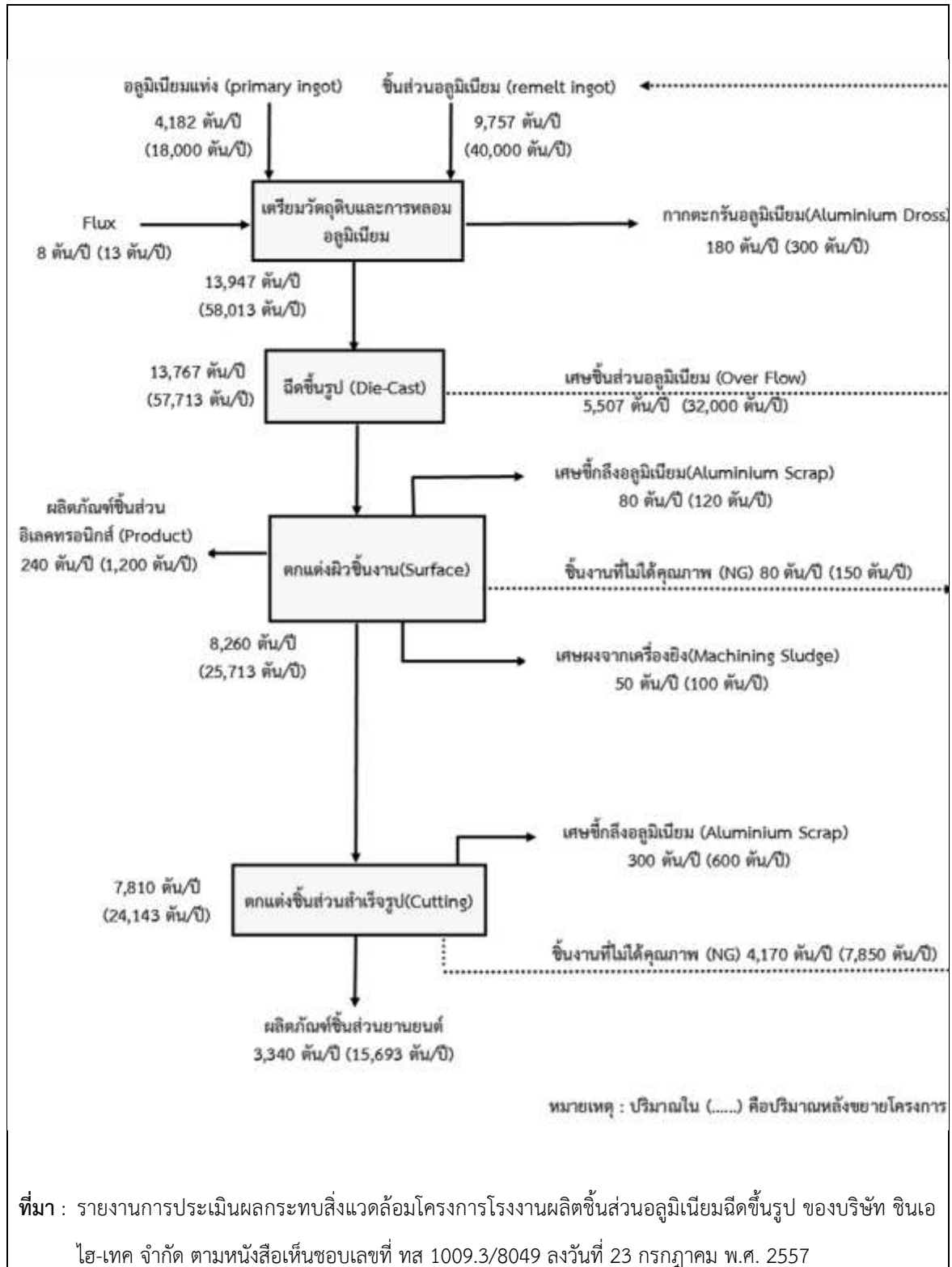
รูปที่ 2.4-1 ผังตุลมวลการผลิตของโครงการ
