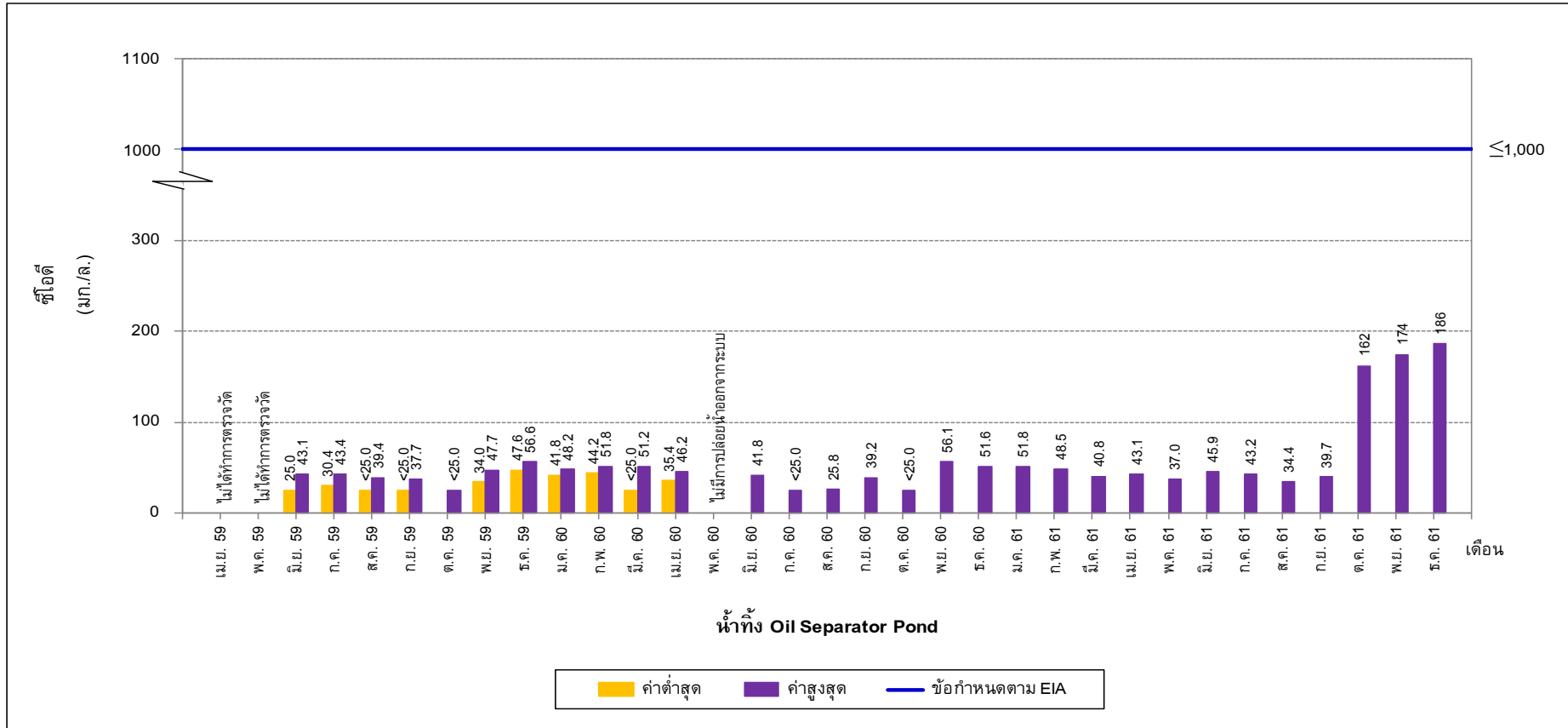
รูปที่ 5-36 เปรียบเทียบซีโอดี ในน้ำทิ้ง Oil Separator Pond ระหว่างปี พ.ศ. 2559-2561
