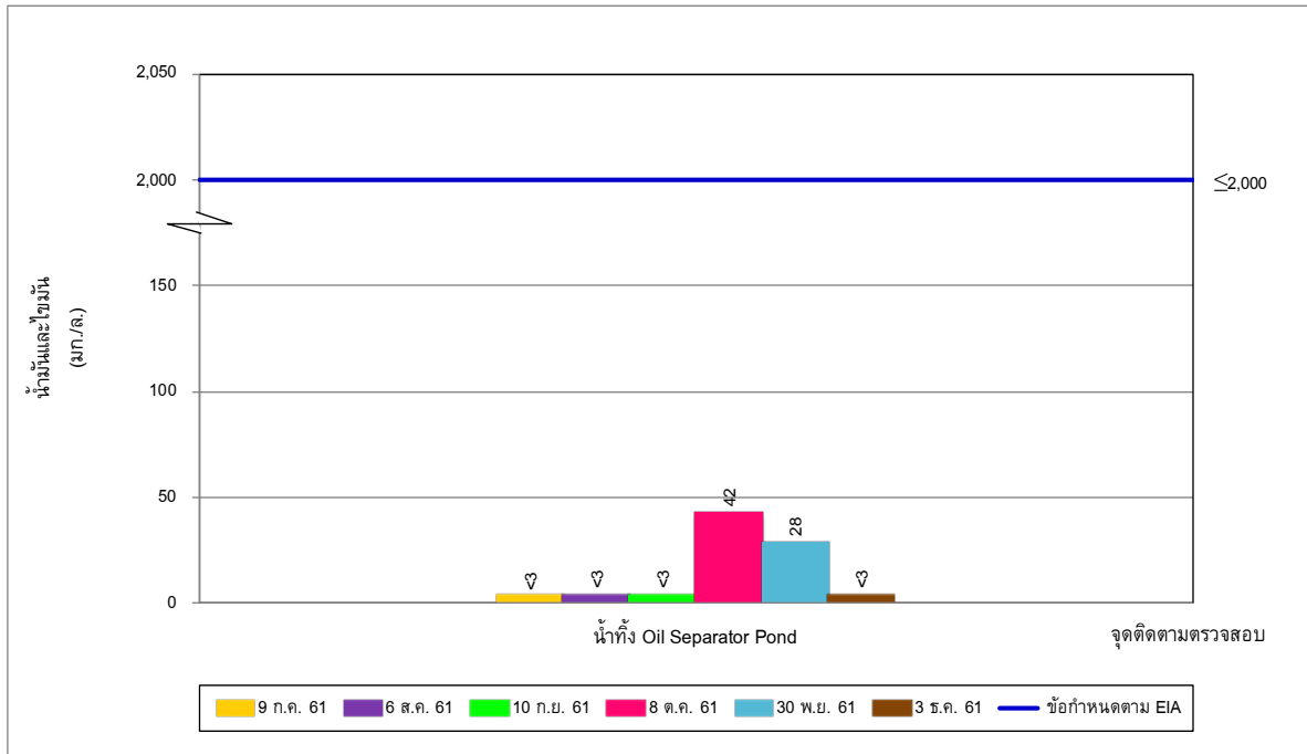
รูปที่ 5-17 ผลการติดตามตรวจสอบน้ำมันและไขมัน ในน้ำทิ้ง Oil Separator Pond ระหว่างเดือนกรกฎาคม-ธันวาคม พ.ศ. 2561
