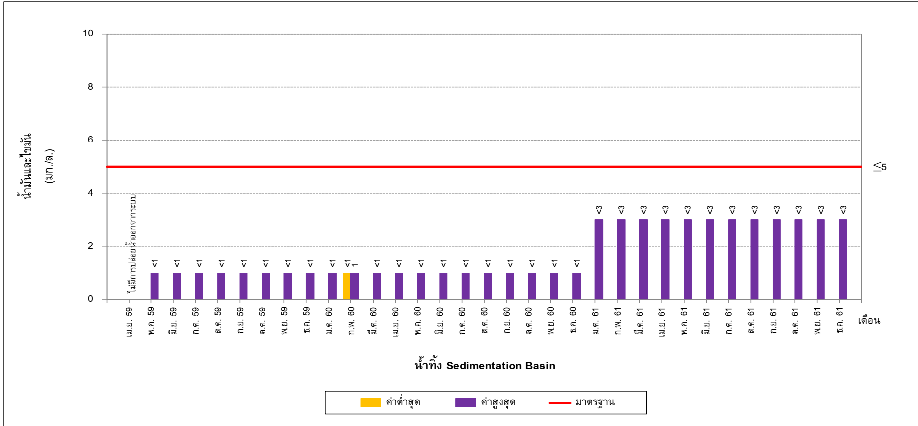
รูปที่ 5-28 เปรียบเทียบน้ำมันและไขมัน ในน้ำทิ้ง Sedimentation Basin ระหว่างปี พ.ศ. 2559-2561
