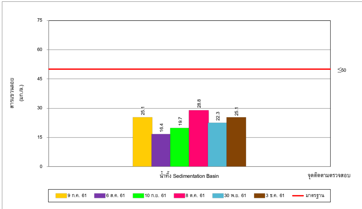
รูปที่ 5-3 ผลการติดตามตรวจสอบสารแขวนลอย ในน้ำทิ้ง Sedimentation Basin ระหว่างเดือนกรกฎาคม-ธันวาคม พ.ศ. 2561
