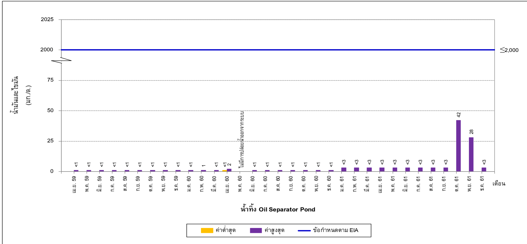
รูปที่ 5-39 เปรียบเทียบน้ำมันและไขมัน ในน้ำทิ้ง Oil Separator Pond ระหว่างปี พ.ศ. 2559-2561
