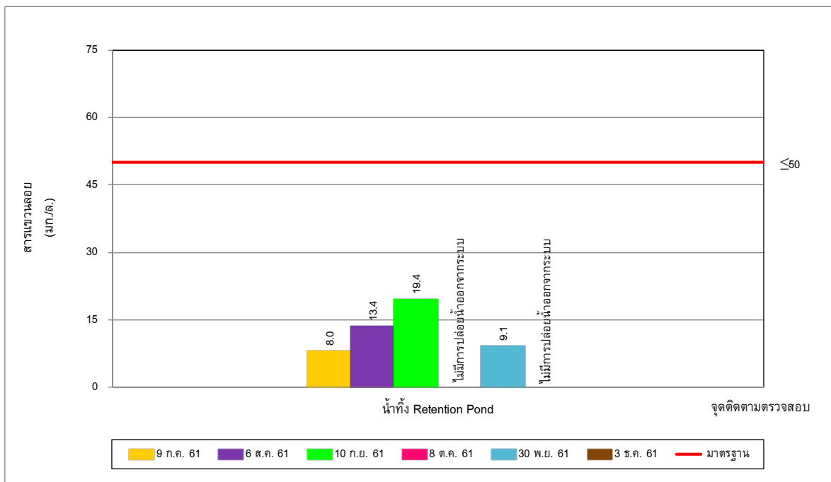
รูปที่ 5-9 ผลการติดตามตรวจสอบสารแขวนลอย ในน้ำทิ้ง Retention Pond ระหว่างเดือนกรกฎาคม-ธันวาคม พ.ศ. 2561
