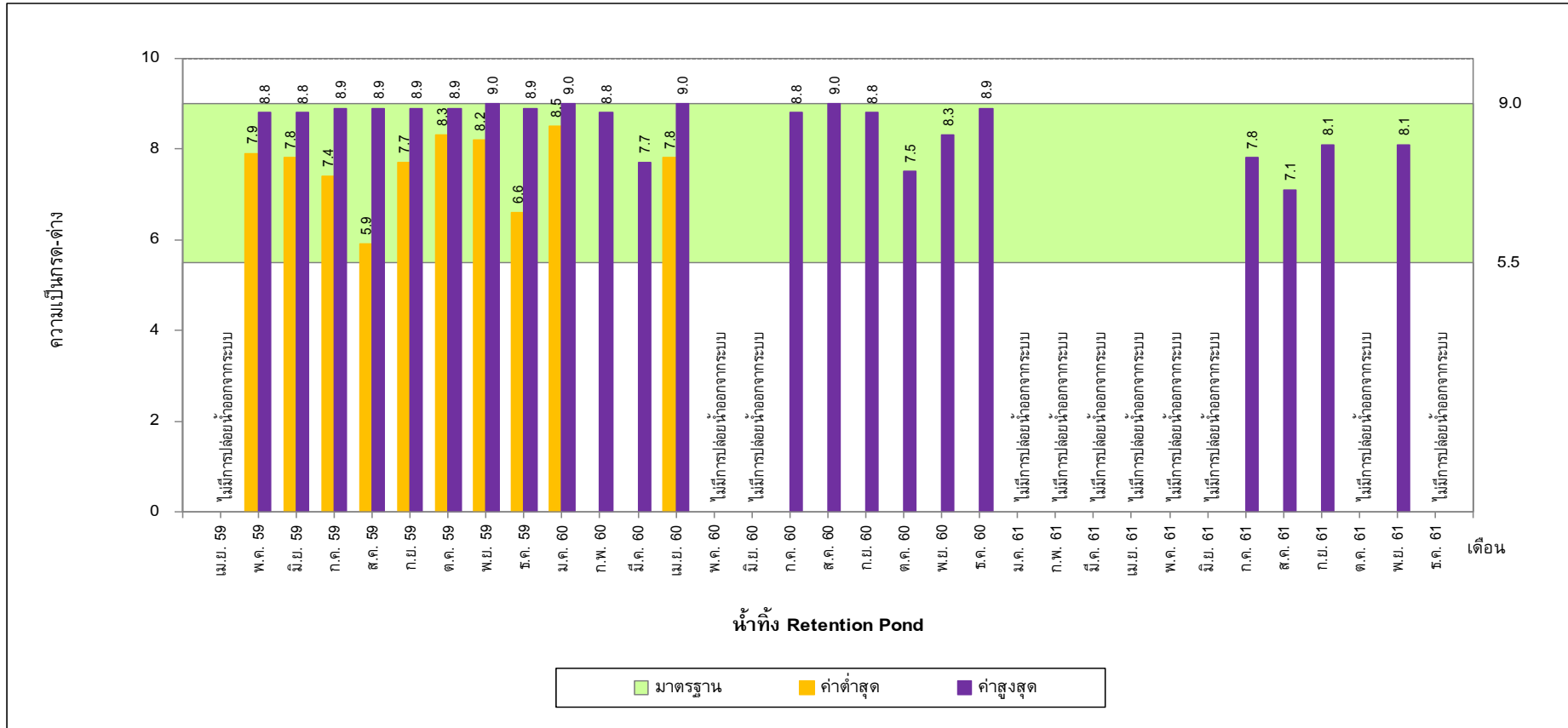
รูปที่ 5-29 เปรียบเทียบความเป็นกรด-ต่าง ในหน้าทิ้ง Retention Pond ระหว่างปี พ.ศ. 2559-2561
