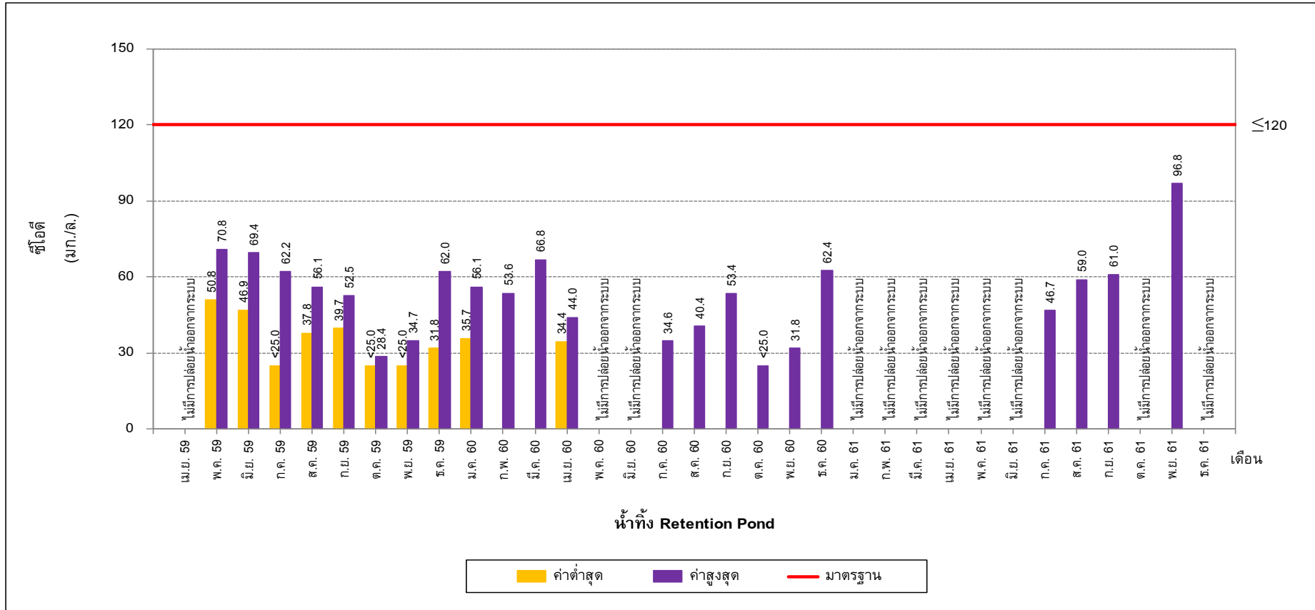
รูปที่ 5-30 เปรียบเทียบซีโอดี ในน้ำทิ้ง Retention Pond ระหว่างปี พ.ศ. 2559-2561
