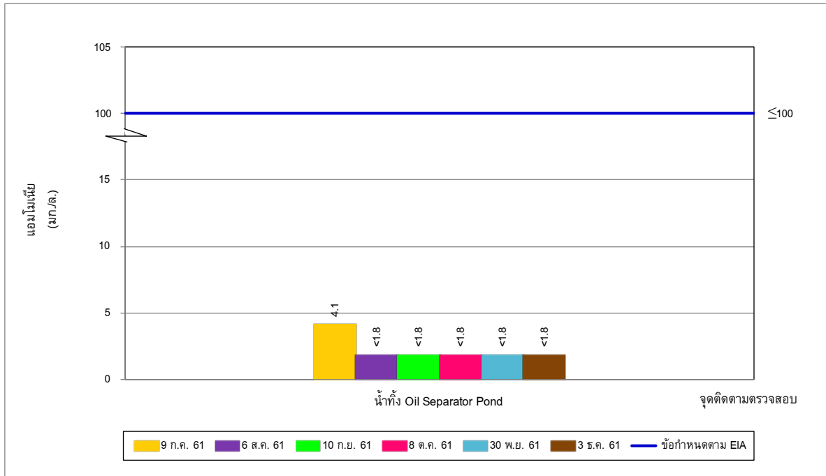
รูปที่ 5-15 ผลการติดตามตรวจสอบแอมโมเนีย ในน้ำทิ้ง Oil Separator Pond ระหว่างเดือนกรกฎาคม-ธันวาคม พ.ศ. 2561
