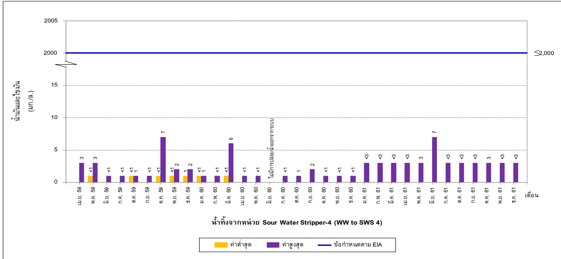
รูปที่ 5-44 เปรียบเทียบน้ำมันและไซนีน ในน้ำทิ้งจากหน่วย Sour Water Stripper-4 (WW to SWS 4) ระหว่างปี พ.ศ. 2559-2561
