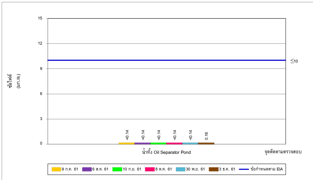
รูปที่ 5-16 ผลการติดตามตรวจสอบคลอไรด์ ในน้ำทิ้ง Oil Separator Pond ระหว่างเดือนกรกฎาคม-ธันวาคม พ.ศ. 2561
