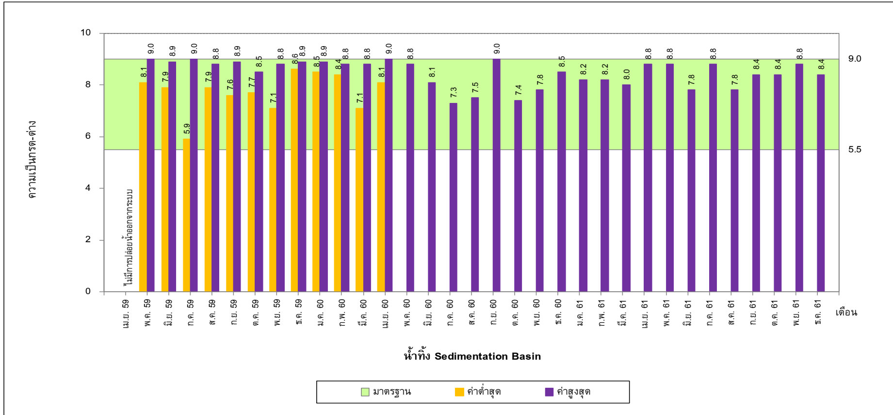
รูปที่ 5-23 เปรียบเทียบความเป็นกรด-ต่าง ในหน้าห้อง Sedimentation Basin ระหว่างปี พ.ศ. 2559-2561
