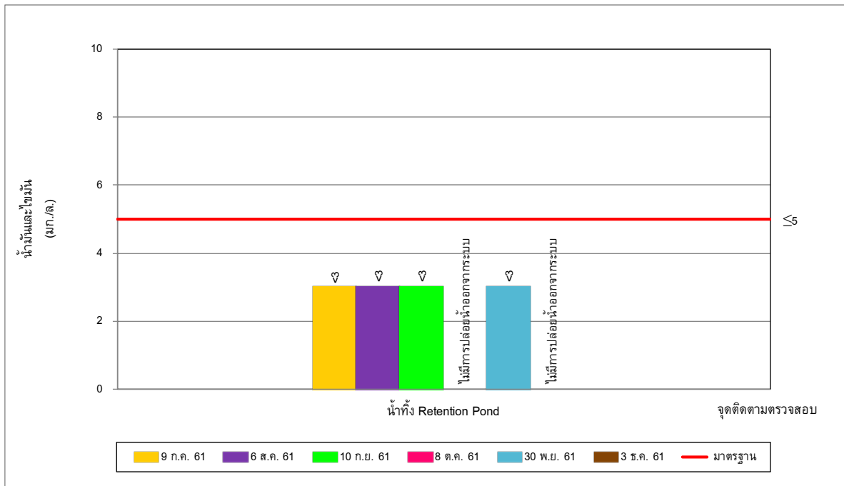
รูปที่ 5-12 ผลการติดตามตรวจสอบแอมโมเนียและไนไตรต์ ในน้ำทิ้ง Retention Pond ระหว่างเดือนกรกฎาคม-ธันวาคม พ.ศ. 2561
