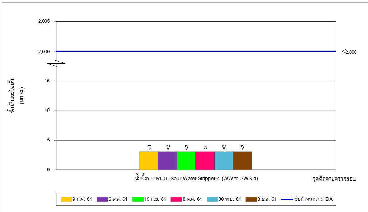
รูปที่ 5-22 ผลการติดตามตรวจสอบน้ำมันและไขมัน ในน้ำทิ้งจากหน่วย Sour Water Stripper-4 (WW to SWS 4) ระหว่างเดือนกรกฎาคม-ธันวาคม พ.ศ. 2561
