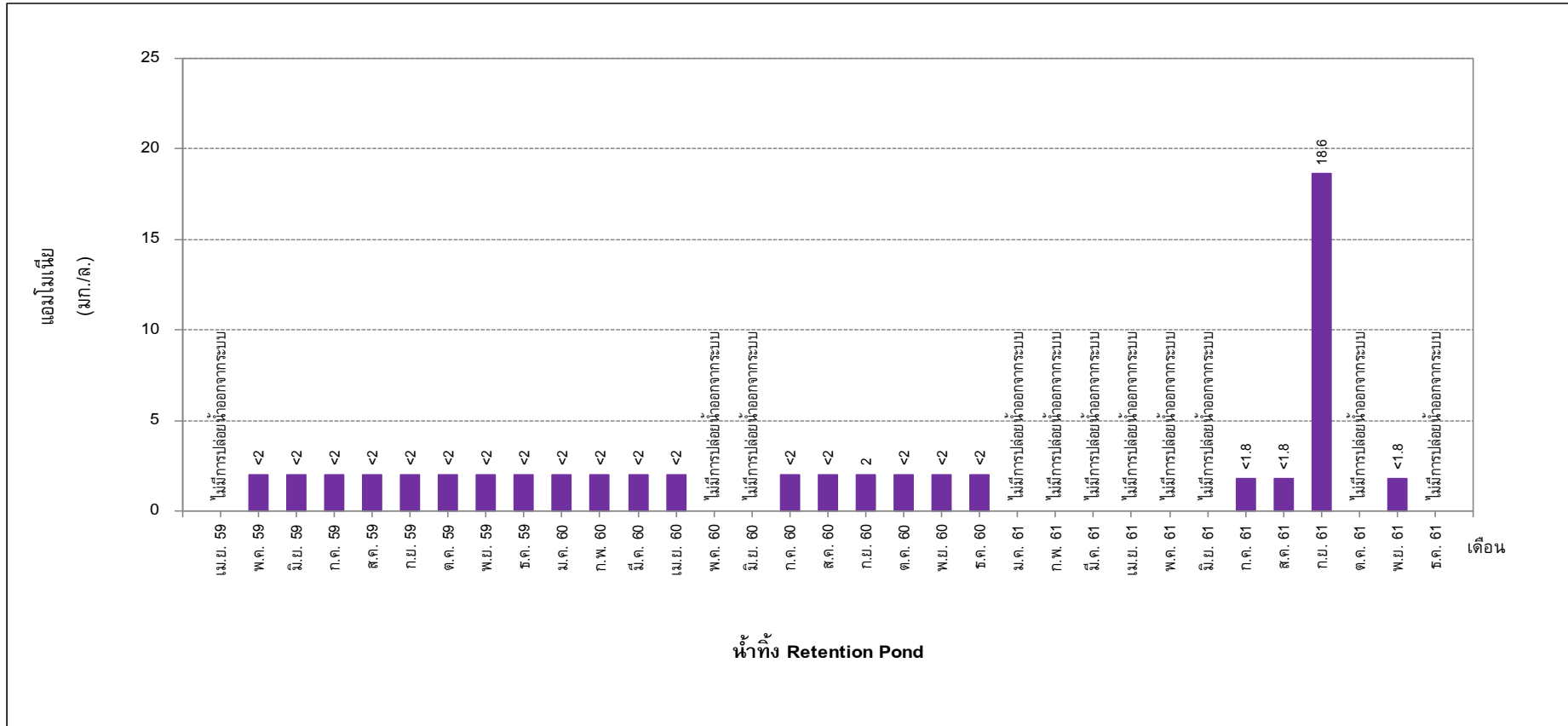
รูปที่ 5-32 เปรียบเทียบแอมโมเนีย ในน้ำทิ้ง Retention Pond ระหว่างปี พ.ศ. 2559-2561
