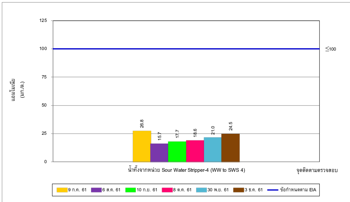
รูปที่ 5-20 ผลการติดตามตรวจสอบแอมโมเนียไนโตรเจนในน้ำทิ้งจากหน่วย Sour Water Stripper-4 (WW to SWS 4) ระหว่างเดือนกรกฎาคม-ธันวาคม พ.ศ. 2561
