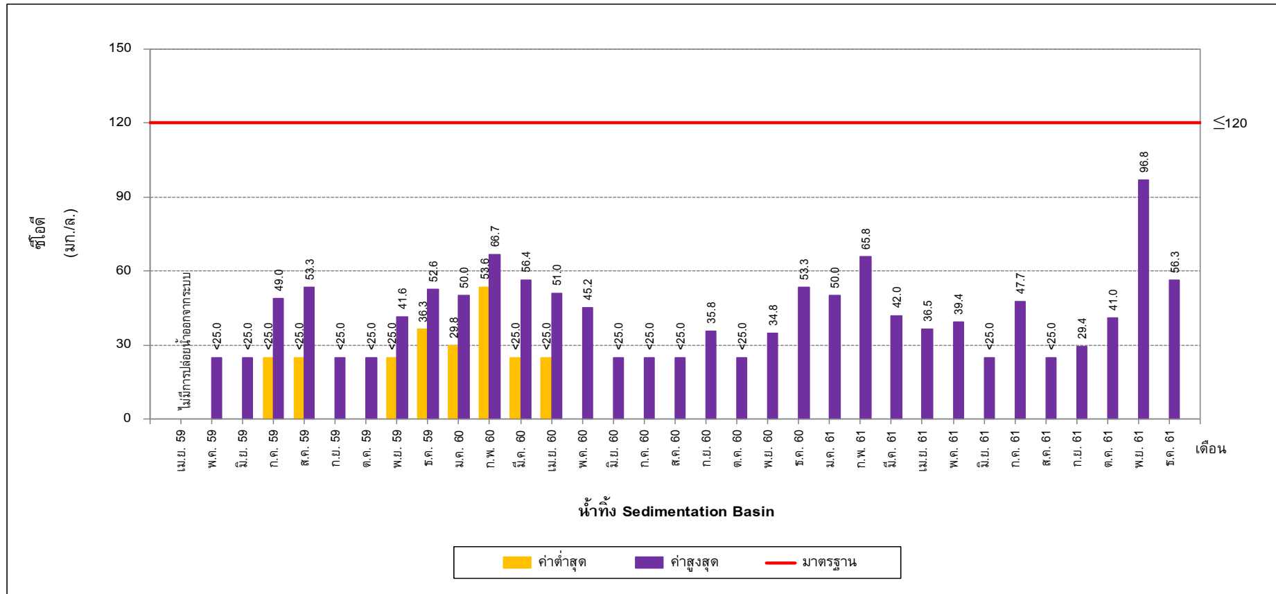
รูปที่ 5-24 เปรียบเทียบซีโอดี ในน้ำทิ้ง Sedimentation Basin ระหว่างปี พ.ศ. 2559-2561
