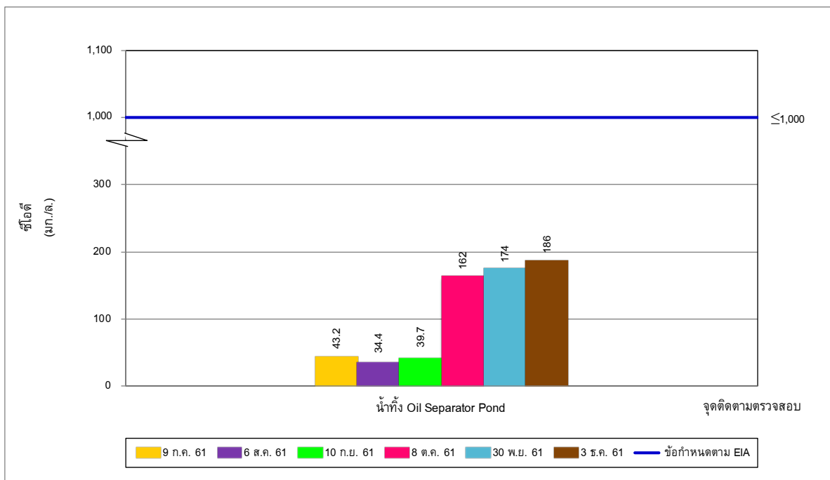
รูปที่ 5-14 ผลการติดตามตรวจสอบซีโอดี ในน้ำทิ้ง Oil Separator Pond ระหว่างเดือนกรกฎาคม-ธันวาคม พ.ศ. 2561
