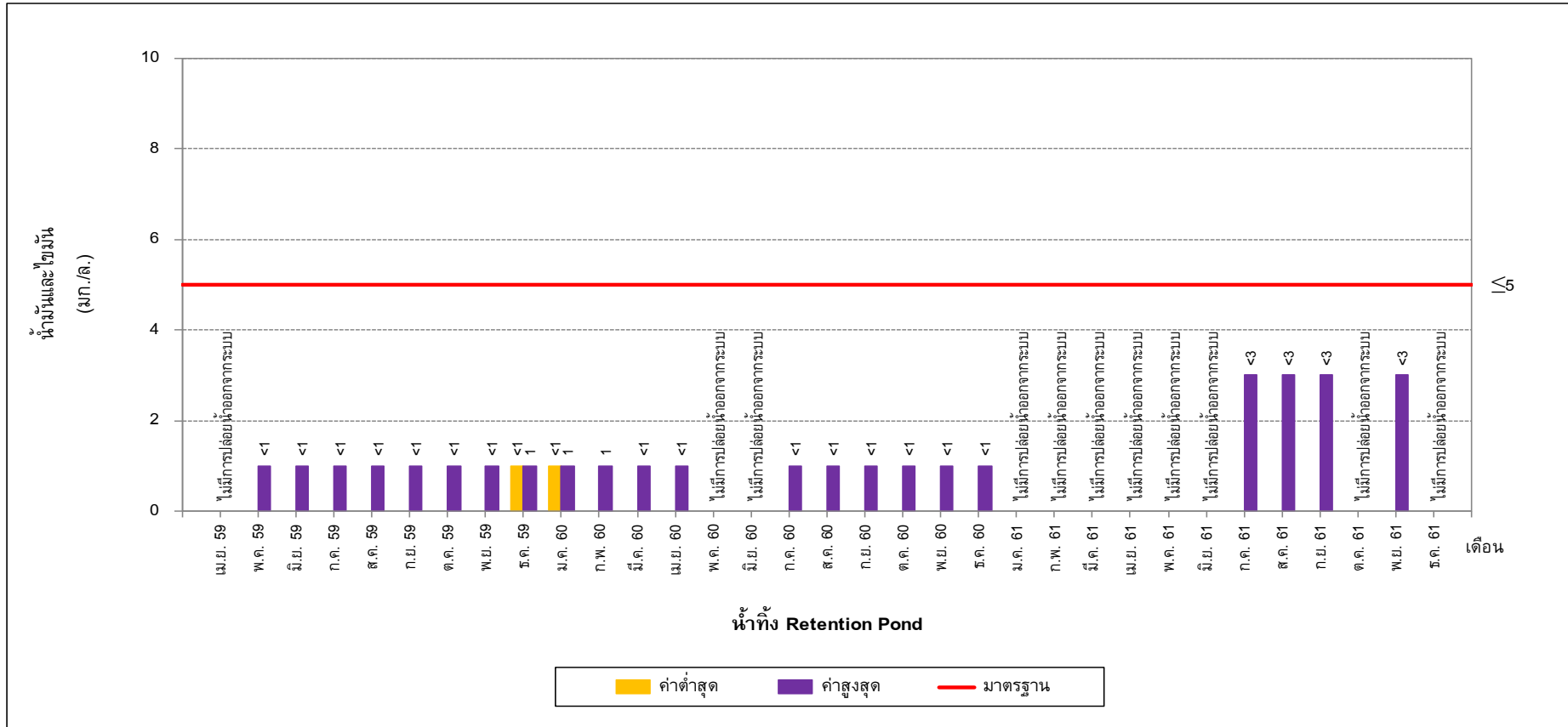
รูปที่ 5-34 เปรียบเทียบน้ำมันและไนโตรเจน ในน้ำทิ้ง Retention Pond ระหว่างปี พ.ศ. 2559-2561
