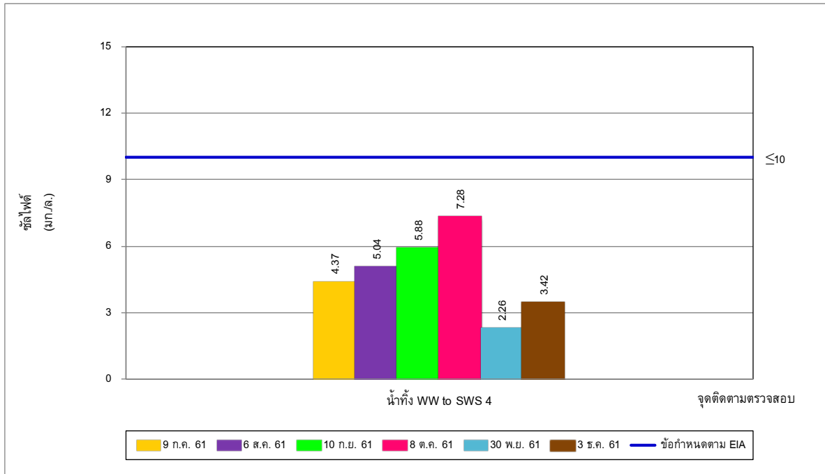
รูปที่ 5-21 ผลการติดตามตรวจสอบซัลไฟด์ ในน้ำทิ้งจากหน่วย Sour Water Stripper-4 (WW to SWS 4) ระหว่างเดือนกรกฎาคม-ธันวาคม พ.ศ. 2561
