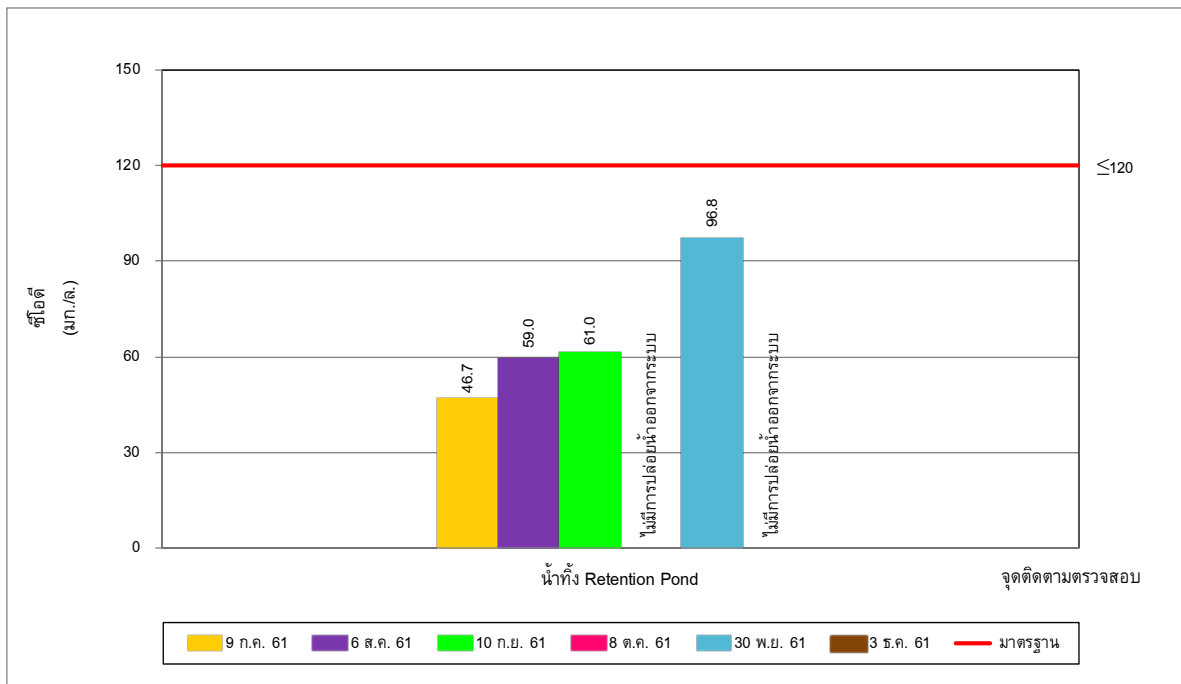
รูปที่ 5-8 ผลการติดตามตรวจสอบซีโอดี ในน้ำทิ้ง Retention Pond ระหว่างเดือนกรกฎาคม-ธันวาคม พ.ศ. 2561
