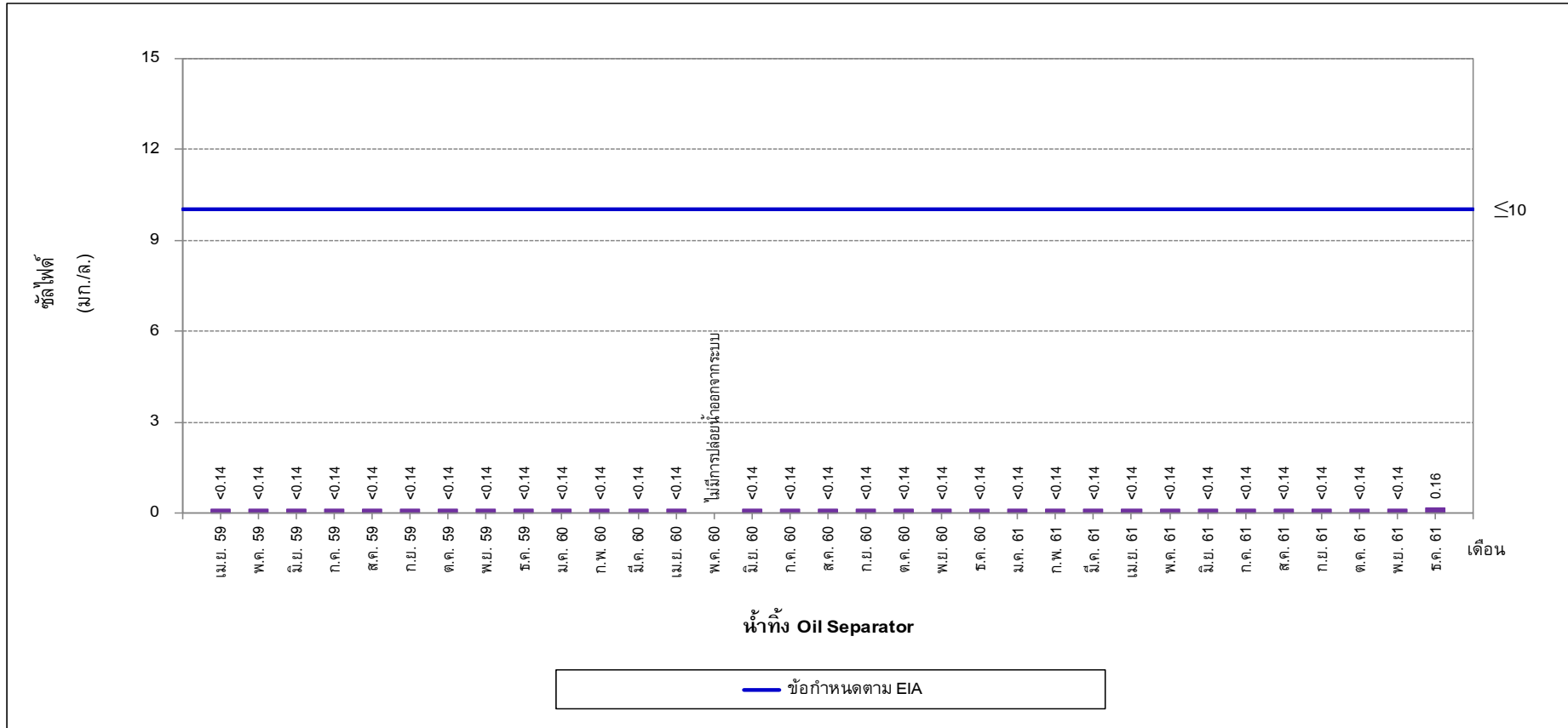
รูปที่ 5-38 เปรียบเทียบซัลไฟด์ในน้ำทิ้ง Oil Separator Pond ระหว่างปี พ.ศ. 2559-2561
