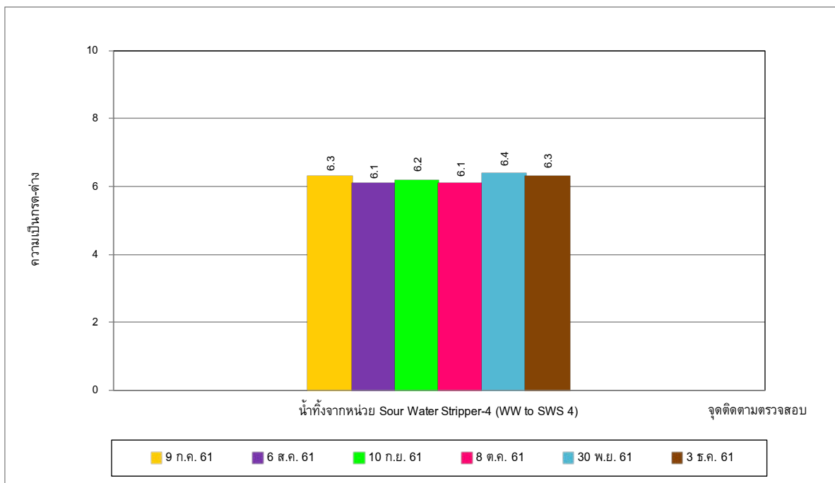
รูปที่ 5-18 ผลการติดตามตรวจสอบความเป็นกรด-ด่าง ในน้ำทิ้งจากหน่วย Sour Water Stripper-4 (WW to SWS 4) ระหว่างเดือนกรกฎาคม-ธันวาคม พ.ศ. 2561
