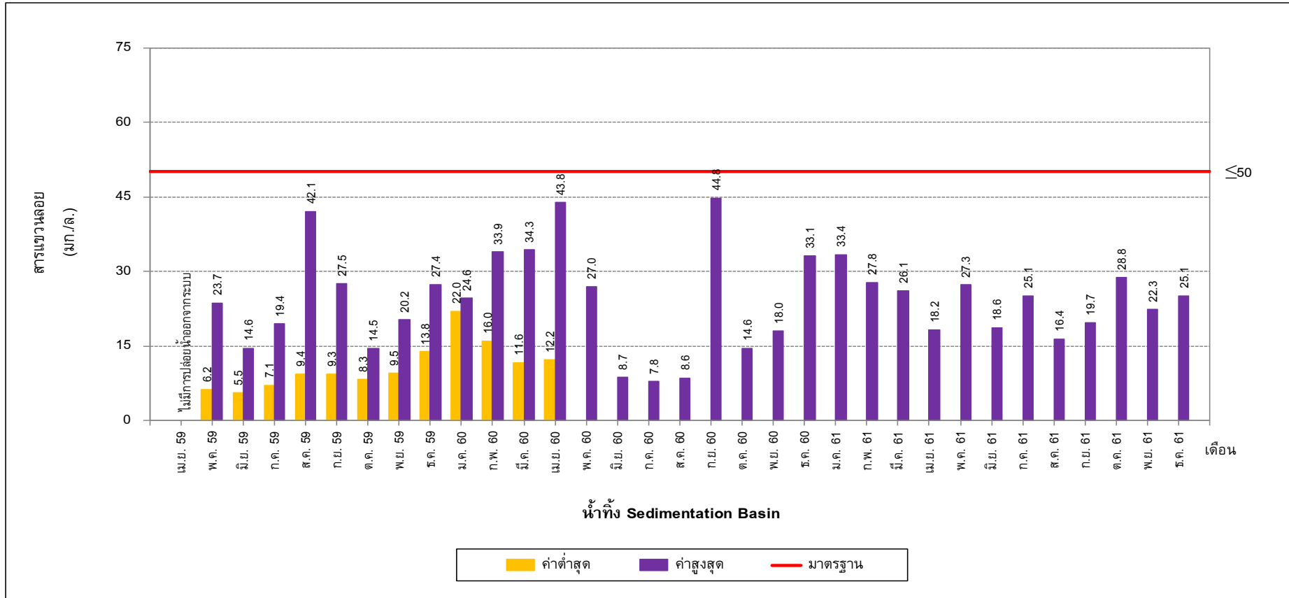
รูปที่ 5-25 เปรียบเทียบสารแขวนลอยในน้ำทิ้ง Sedimentation Basin ระหว่างปี พ.ศ. 2559-2561
