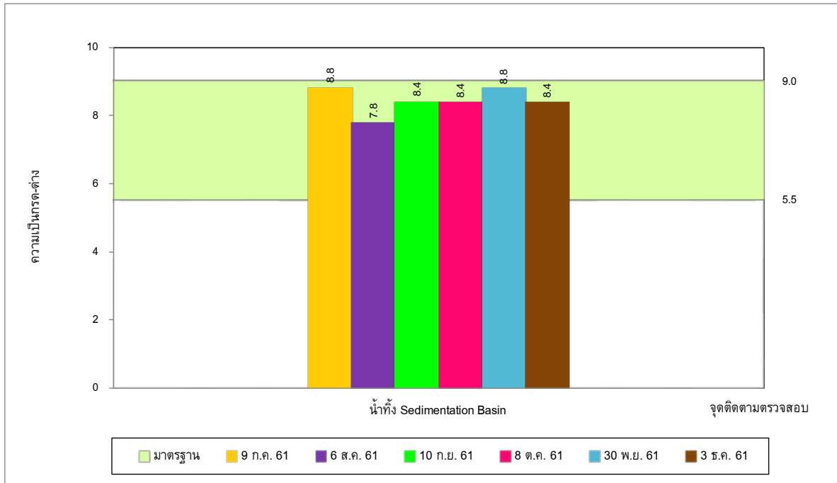
รูปที่ 5-1 ผลการติดตามตรวจสอบความเป็นกรด-ด่าง ในน้ำทิ้ง Sedimentation Basin ระหว่างเดือนกรกฎาคม-ธันวาคม พ.ศ. 2561
