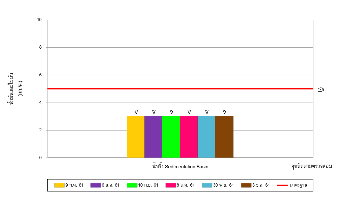
รูปที่ 5-6 ผลการติดตามตรวจสอบน้ำมันและไขมัน ในน้ำทิ้ง Sedimentation Basin ระหว่างเดือนกรกฎาคม-ธันวาคม พ.ศ. 2561
