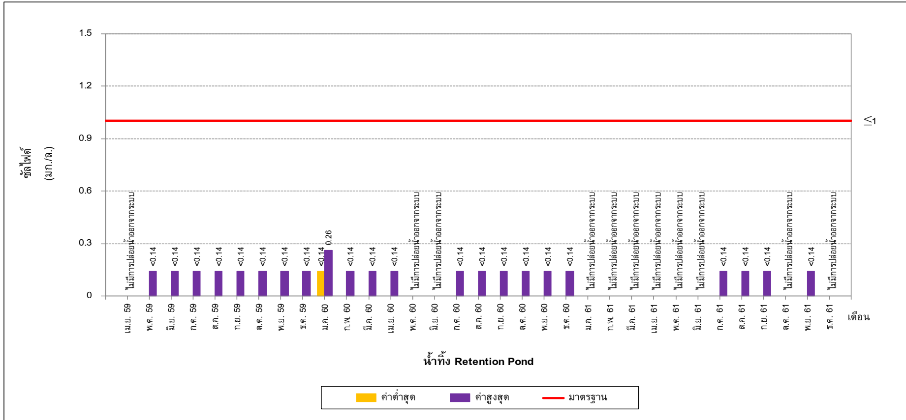
รูปที่ 5-33 เปรียบเทียบชัลไฟต์ในน้ำทั้ง Retention Pond ระหว่างปี พ.ศ. 2559-2561
