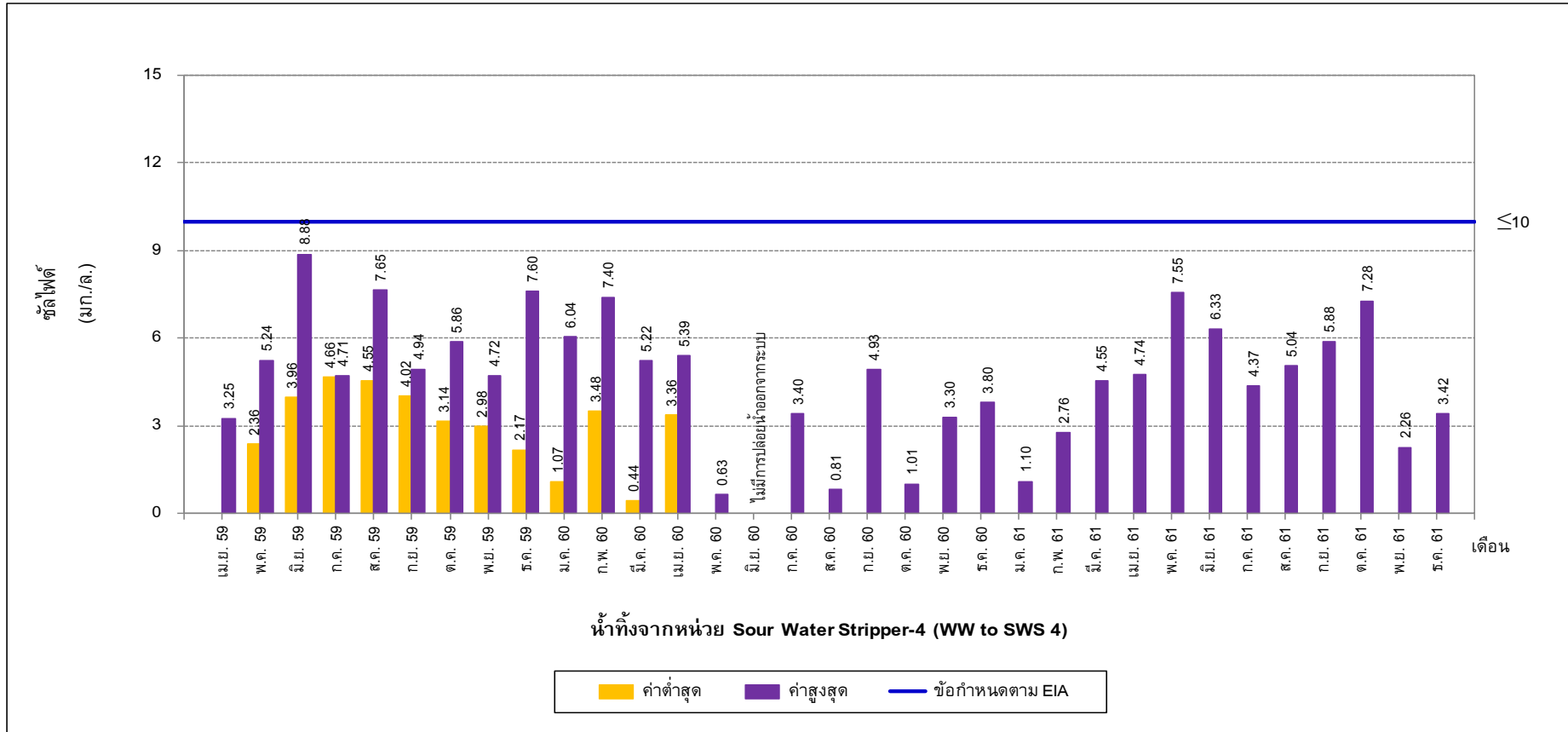
รูปที่ 5-43 เปรียบเทียบซัลไฟด์ในน้ำทิ้งจากหน่วย Sour Water Stripper-4 (WW to SWS 4) ระหว่างปี พ.ศ. 2559-2561
