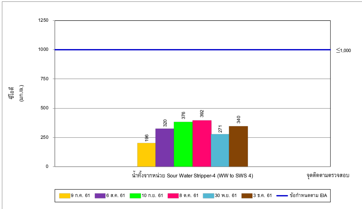
รูปที่ 5-19 ผลการติดตามตรวจสอบซัลเฟตในน้ำทิ้งจากหน่วย Sour Water Stripper-4 (WW to SWS 4) ระหว่างเดือนกรกฎาคม-ธันวาคม พ.ศ. 2561
