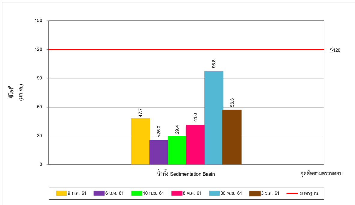
รูปที่ 5-2 ผลการติดตามตรวจสอบซีโอไซด์ ในน้ำทิ้ง Sedimentation Basin ระหว่างเดือนกรกฎาคม-ธันวาคม พ.ศ. 2561
