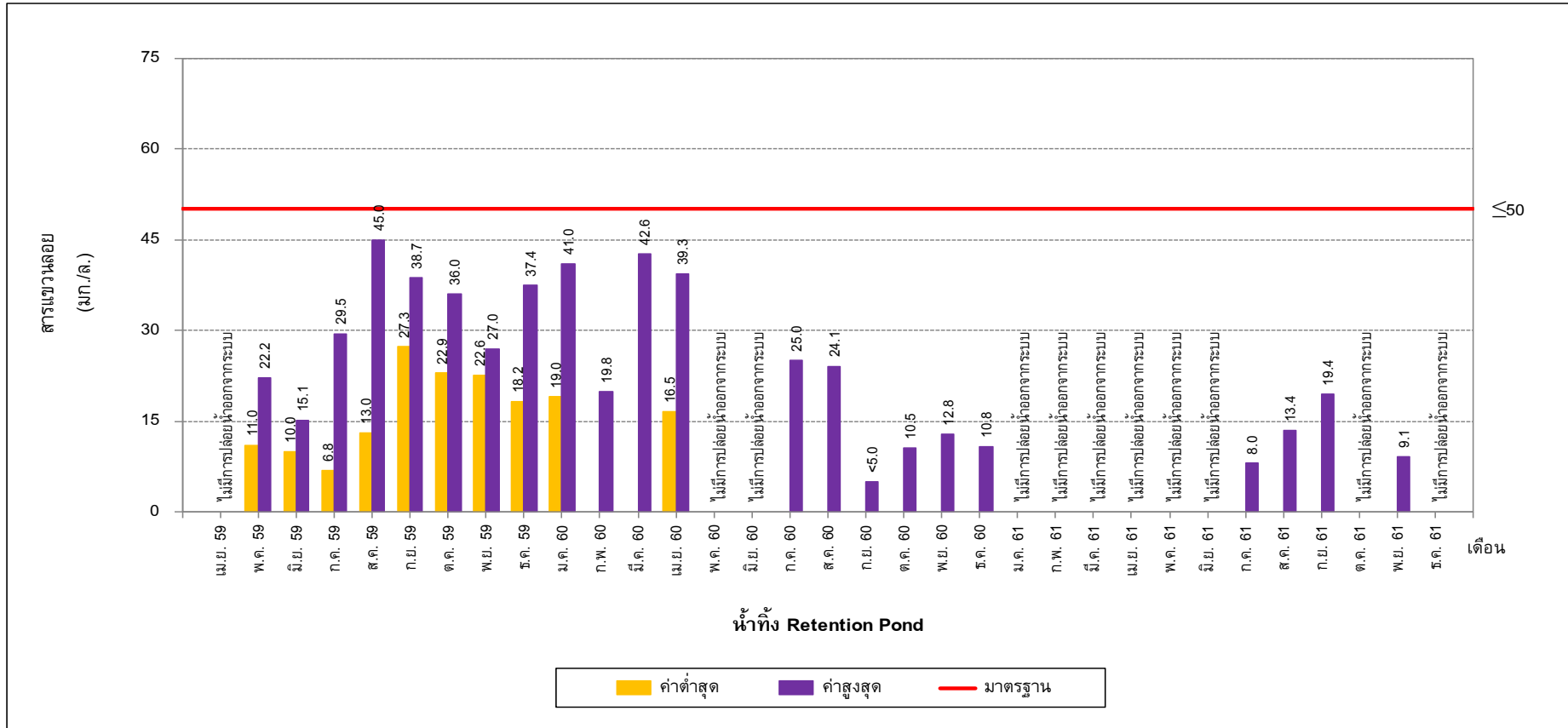
รูปที่ 5-31 เปรียบเทียบสารแขวนลอย ในน้ำทิ้ง Retention Pond ระหว่างปี พ.ศ. 2559-2561
