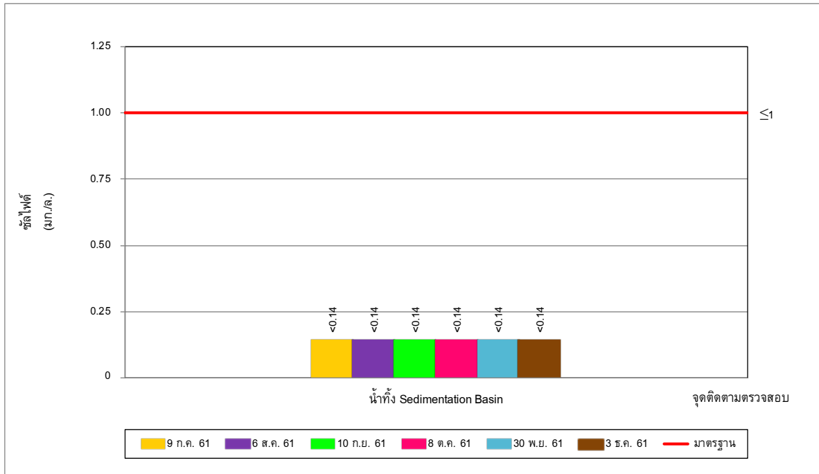
รูปที่ 5-5 ผลการติดตามตรวจสอบซัลไฟด์ ในน้ำทิ้ง Sedimentation Basin ระหว่างเดือนกรกฎาคม-ธันวาคม พ.ศ. 2561
